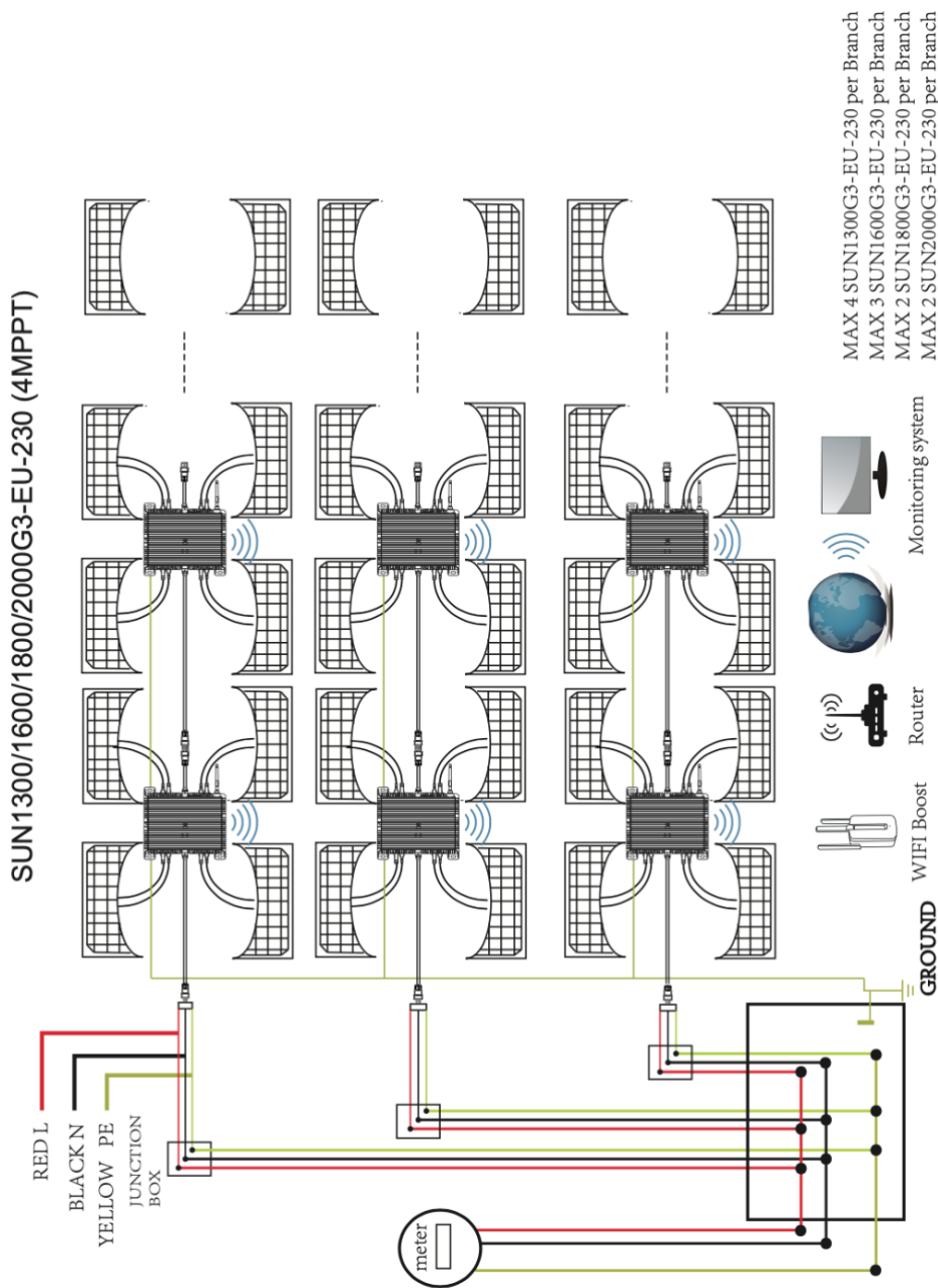
Beispielschaltplan einphasig
