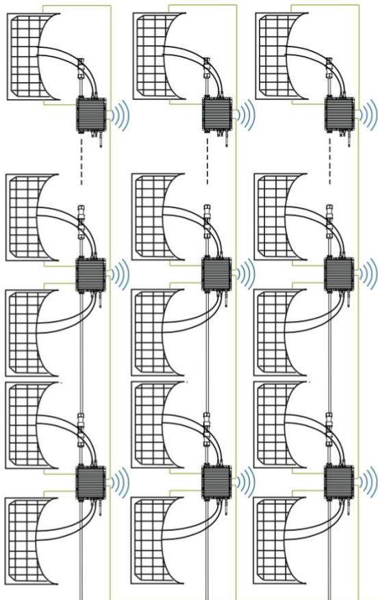
Beispielschaltplan einphasig
